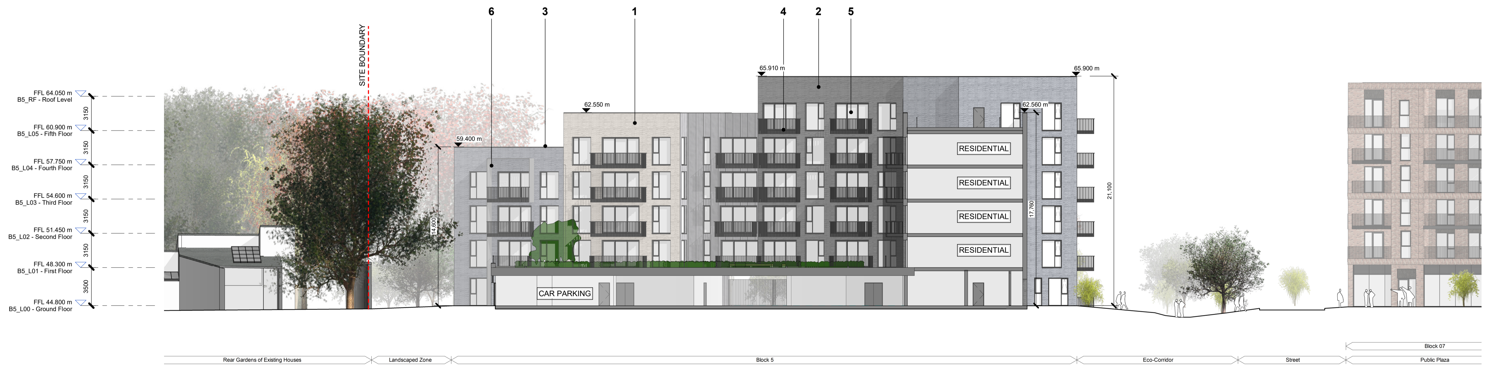
Block 05, N/S Section 02 1 : 200
